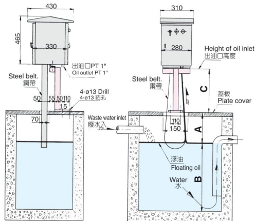
JF-50尺寸圖
