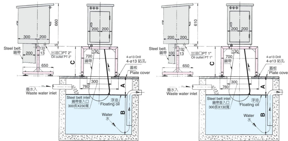
JF-50尺寸圖
